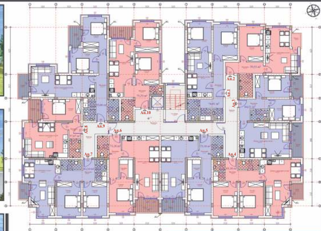
ЕТАЖ - кота +2,63
