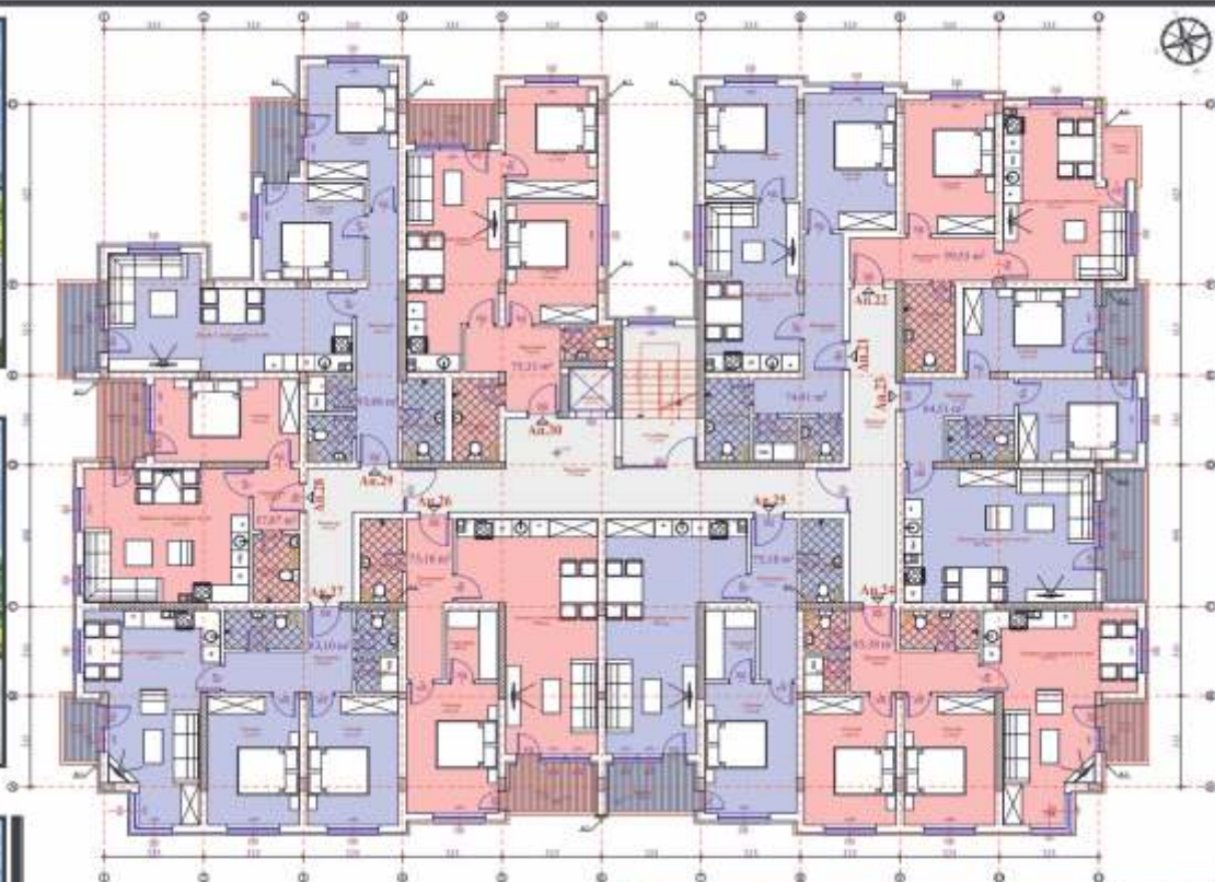
ЕТАЖ IV - кота +8,29
