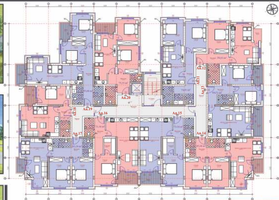
ЕТАЖ III - кота +5,46
