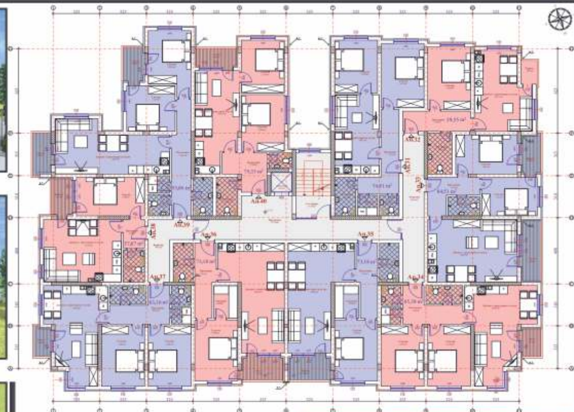
ЕТАЖ V - кота +11,12
