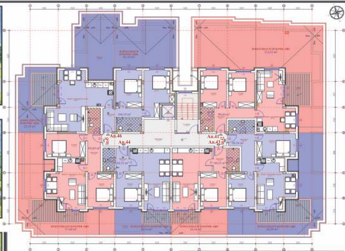
ЕТАЖ VI - кота +13,95
